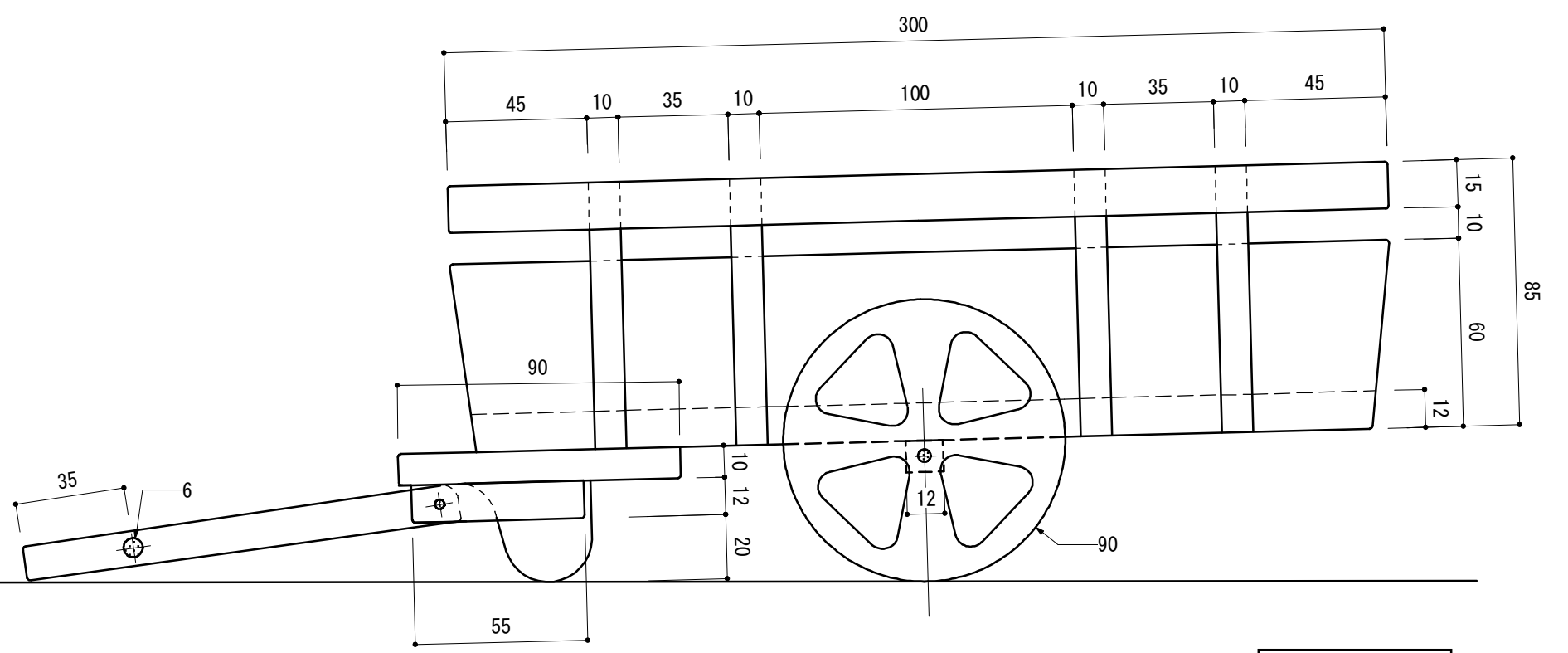
側面図 S:1/2mm
