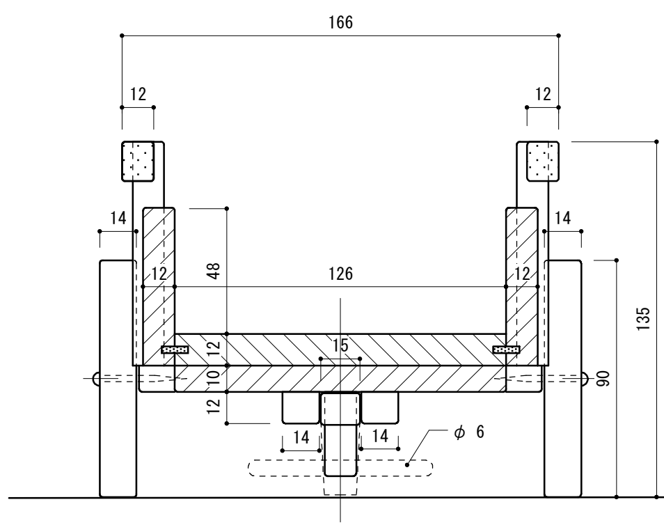
正面図 S:1/2mm
