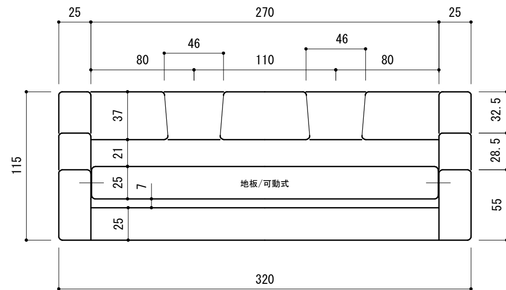
正面図 S:1/3mm
