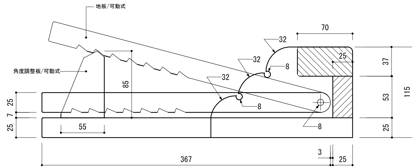
側面図 S:1/3mm
