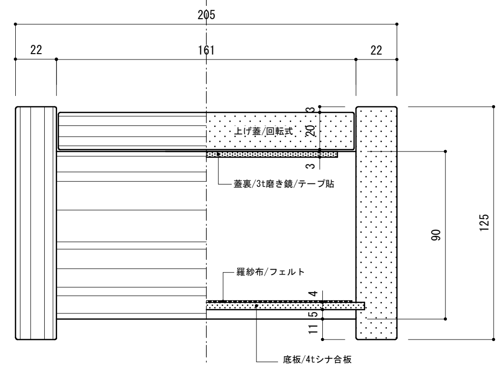
正面図 S:1/2mm
